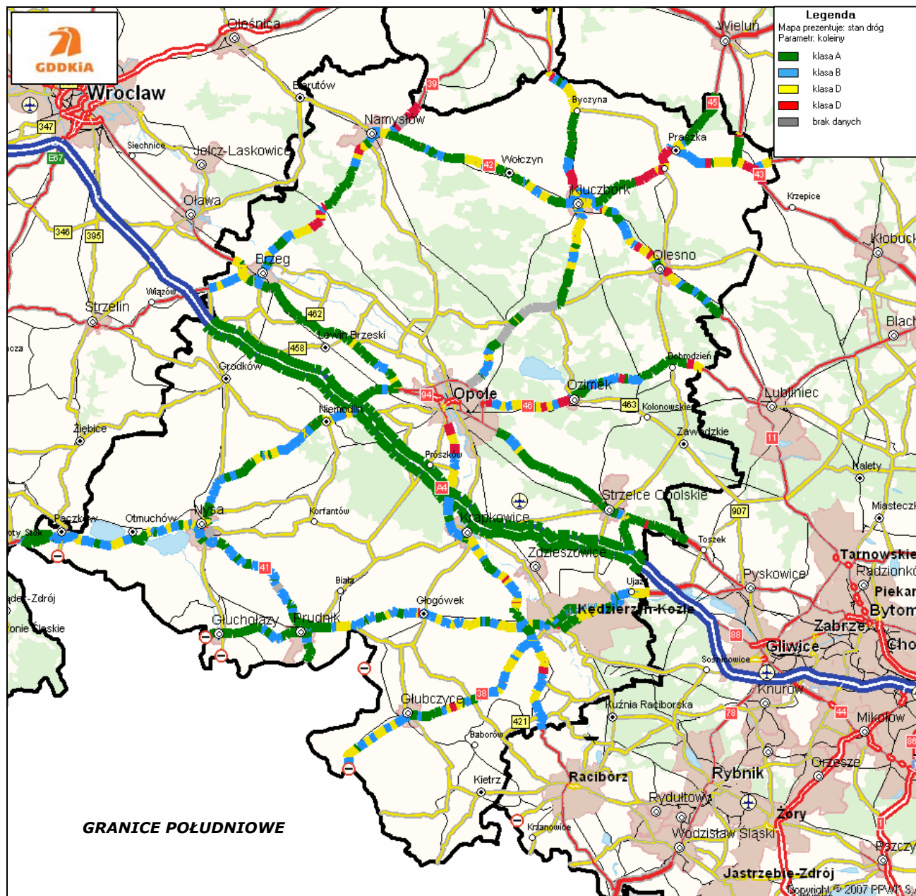
Rysunek 10. Lokalizacja odcinków z koleinami w różnych klasach technicznych na terenie Oddziału w Opolu
