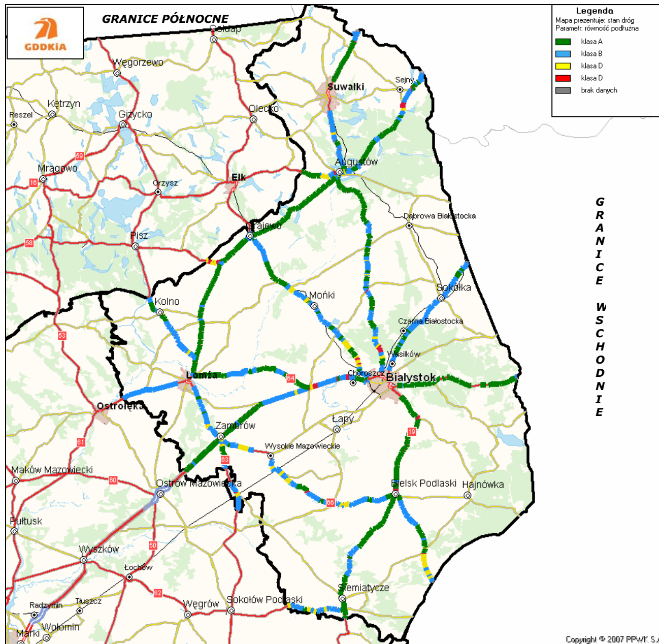
Rysunek 17. Lokalizacja odcinków z równością podłużną w różnych klasach technicznych na terenie Oddziału w Białymstoku
