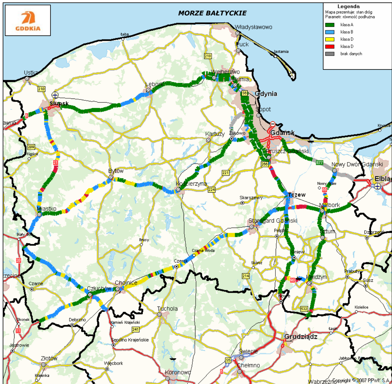
Rysunek 19. Lokalizacja odcinków z równością podłużną w różnych klasach technicznych na terenie Oddziału w Gdańsku
