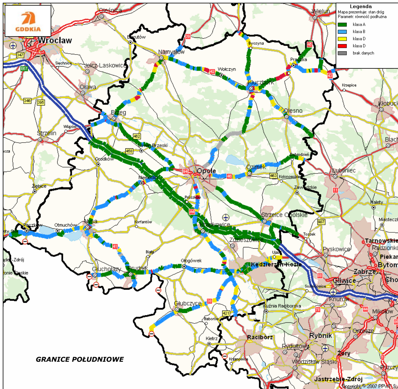
Rysunek 26. Lokalizacja odcinków z równością podłużną w różnych klasach technicznych na terenie Oddziału w Opolu
