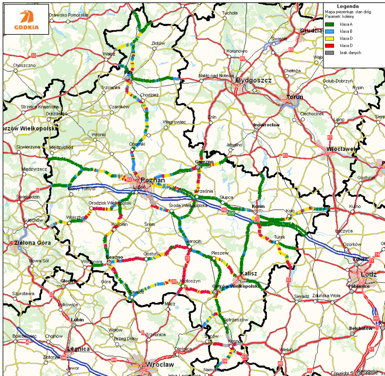
Rysunek 11. Lokalizacja odcinków z koleinami w różnych klasach technicznych na terenie Oddziału w Poznaniu
