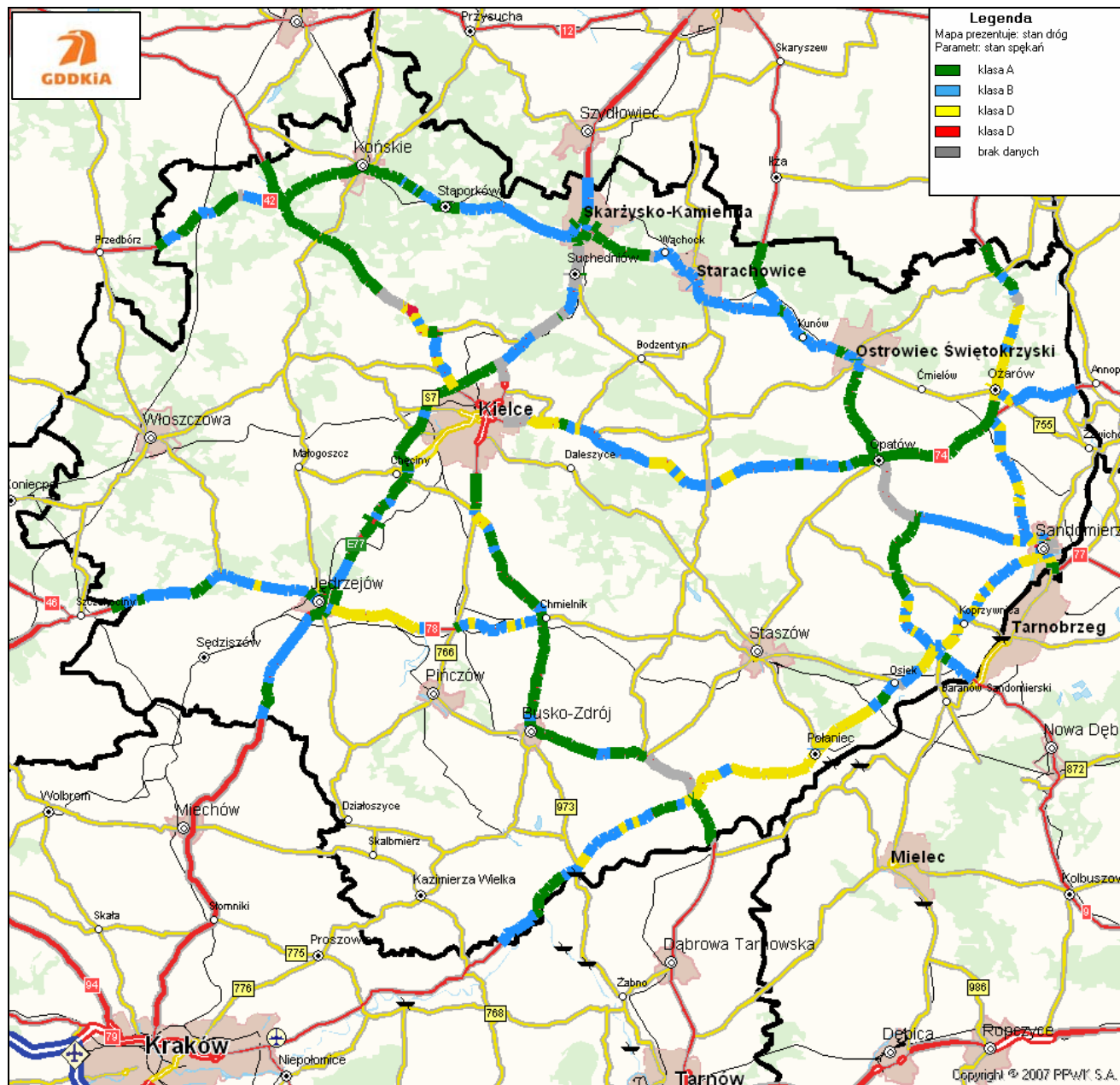
Rysunek 37. Lokalizacja odcinków ze stanem spełnień w różnych klasach technicznych na terenie Oddziału w Kielcach
