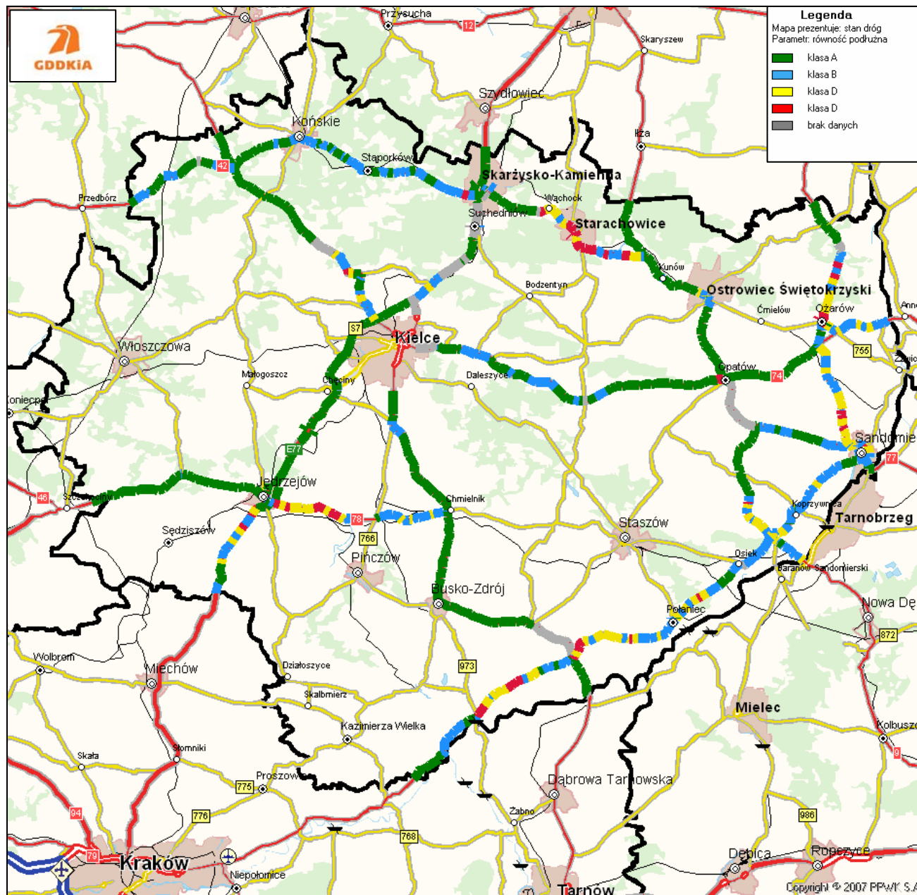
Rysunek 21. Lokalizacja odcinków z równością podłużną w różnych klasach technicznych na terenie Oddziału w Kielcach
