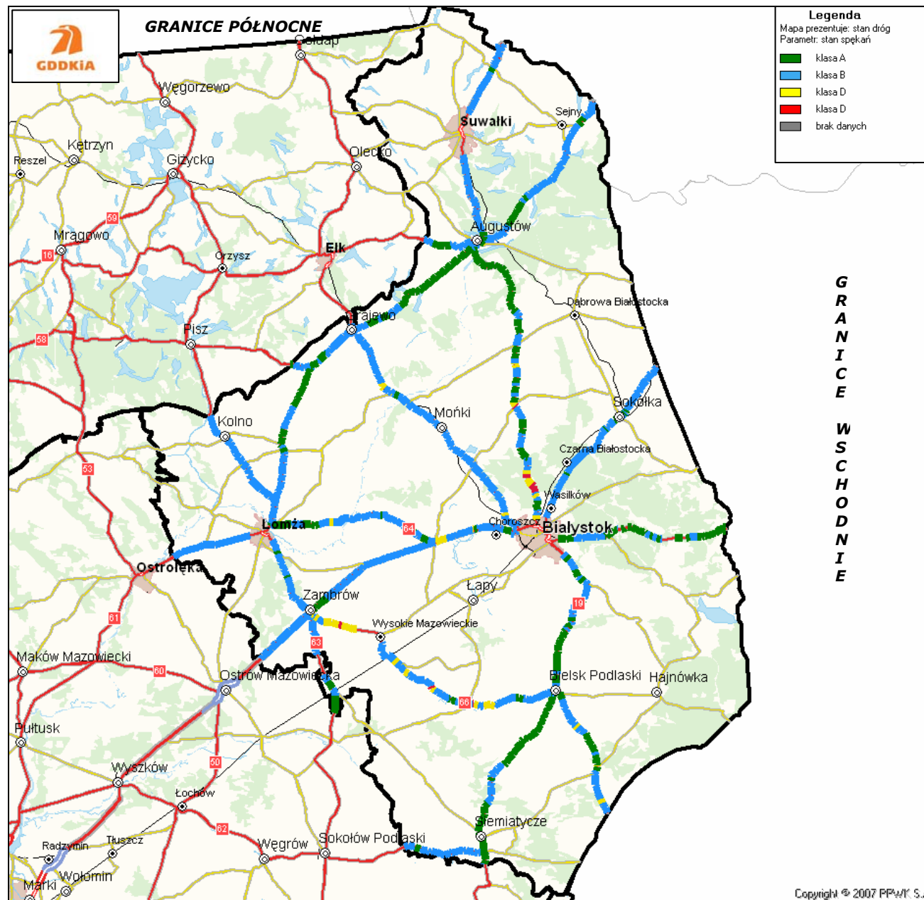
Rysunek 33. Lokalizacja odcinków ze stanem spekań w różnych klasach technicznych na terenie Oddziału w Białymstoku
