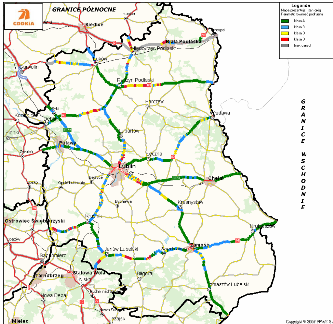
Rysunek 23. Lokalizacja odcinków z równością podłużną w różnych klasach technicznych na terenie Oddziału w Lublinie
