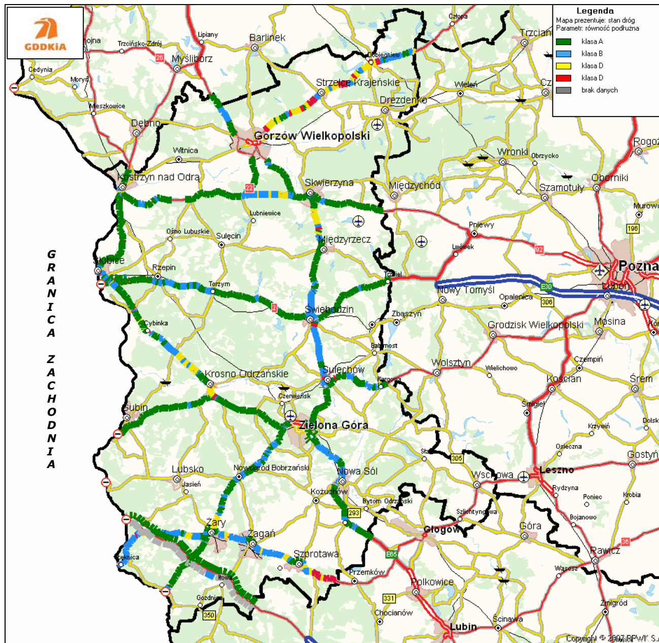
Rysunek 32. Lokalizacja odcinków z równością podłużną w różnych klasach technicznych na terenie Oddziału w Zielonej Górze
