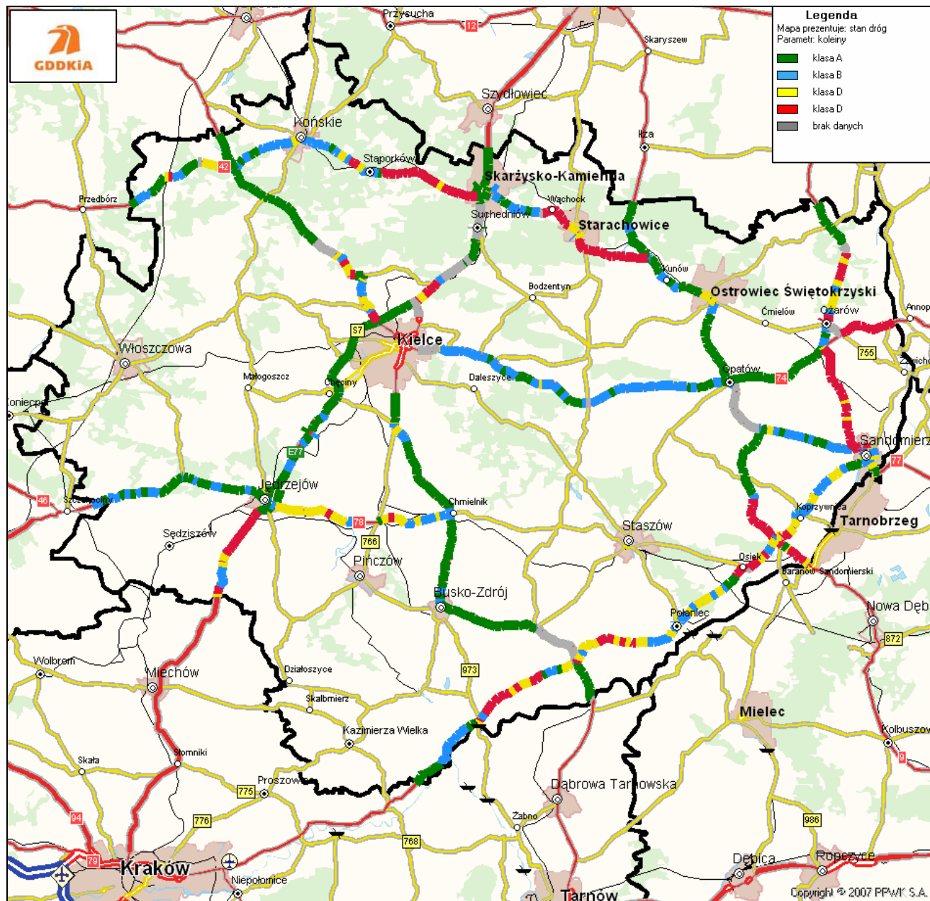
Rysunek 5. Lokalizacja odcinków z kolejniami w różnych klasach technicznych na terenie Oddziału w Kielcach
