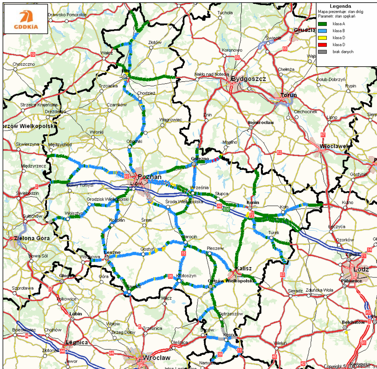
Rysunek 43. Lokalizacja odcinków ze stanem spekań w różnych klasach technicznych na terenie Oddziału w Poznaniu
