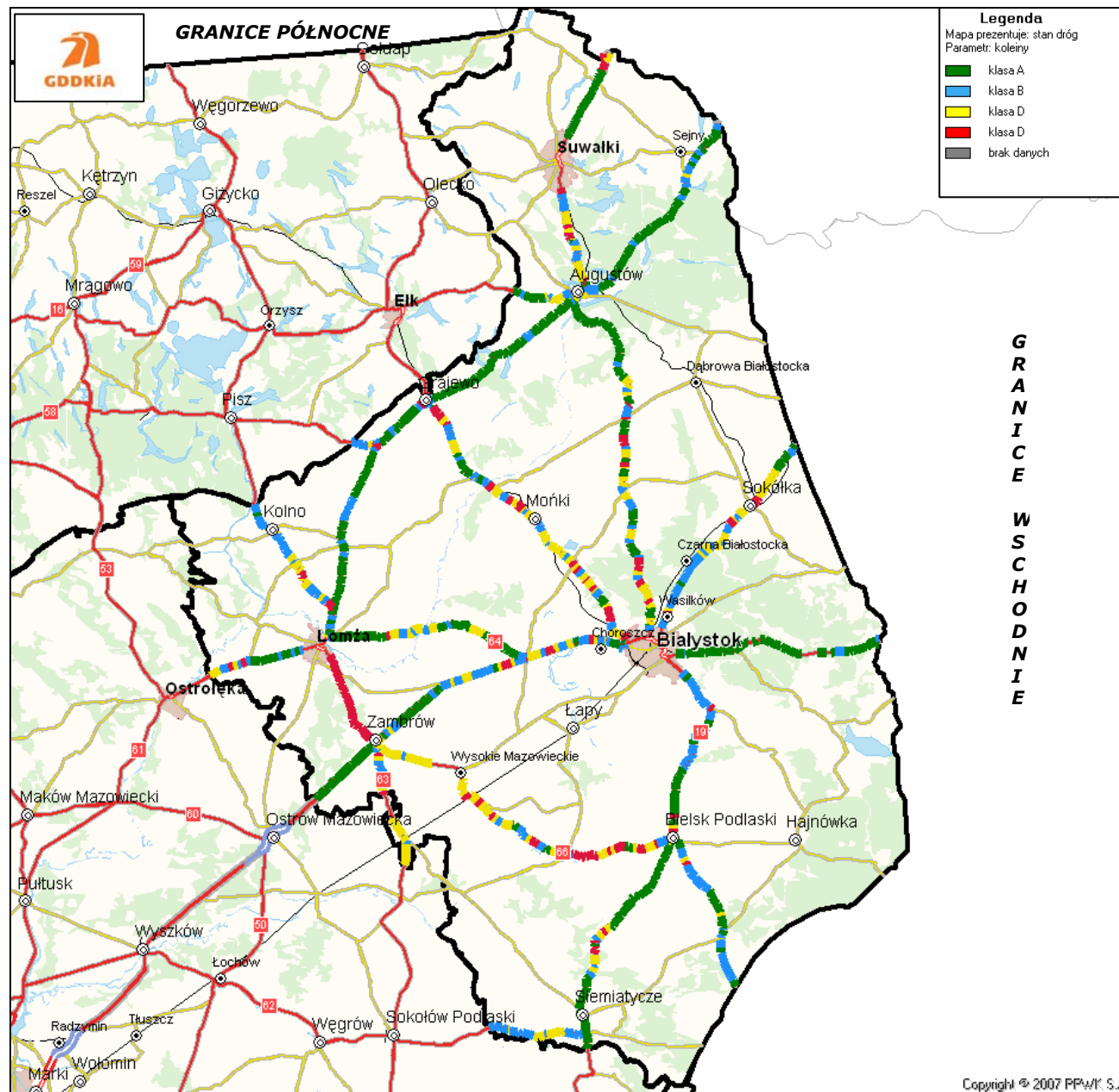
Rysunek 1. Lokalizacja odcinków z koleinami w różnych klasach technicznych na terenie Oddziału w Białymstoku
