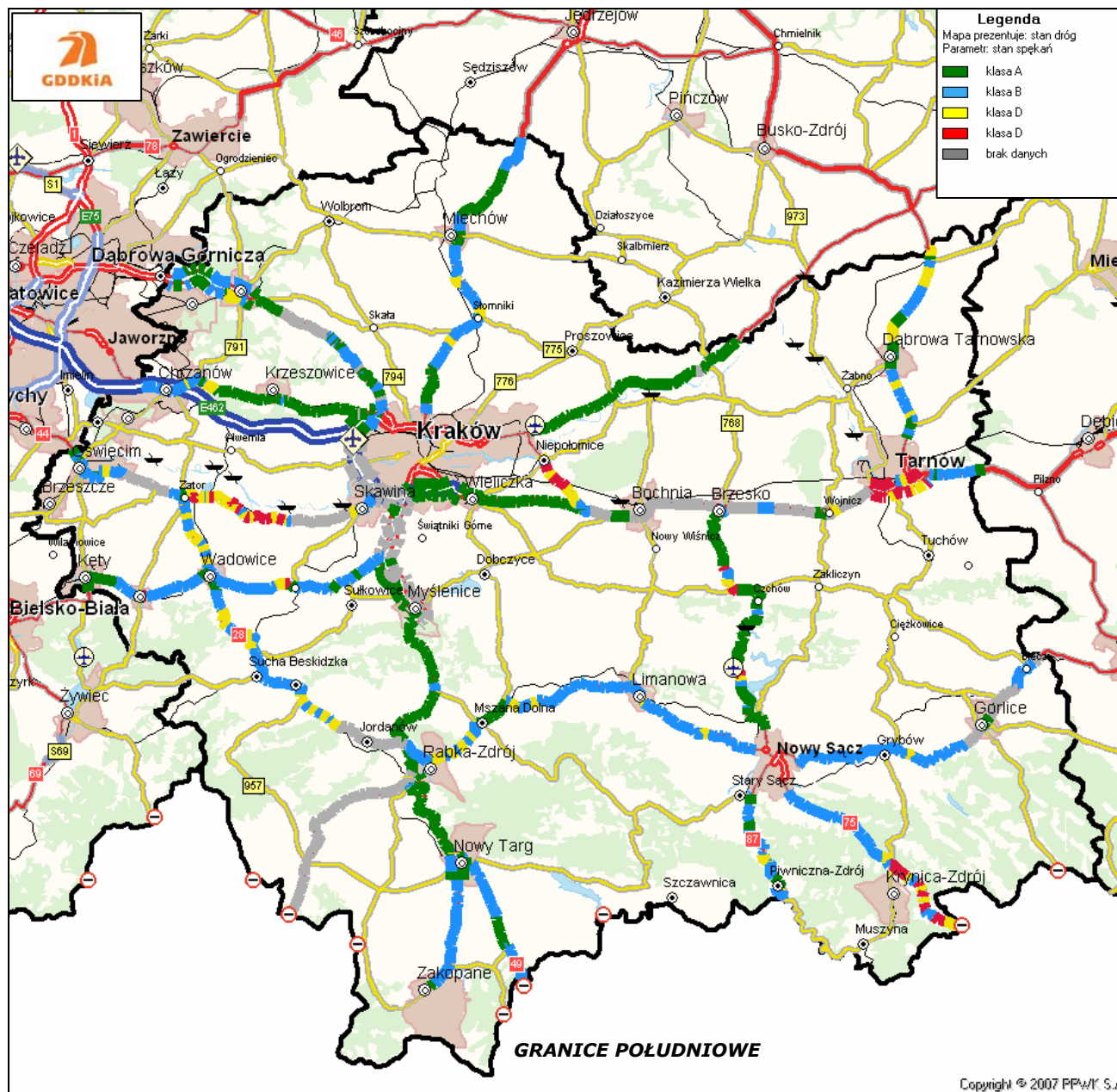
Rysunek 38. Lokalizacja odcinków ze stanem spekań w różnych klasach technicznych na terenie Oddziału w Krakowie
