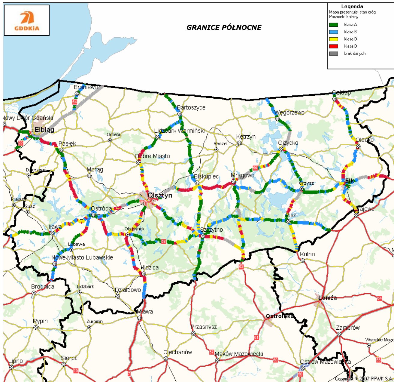
Rysunek 9. Lokalizacja odcinków z kolejniami w różnych klasach technicznych na terenie Oddziału w Olsztynie
