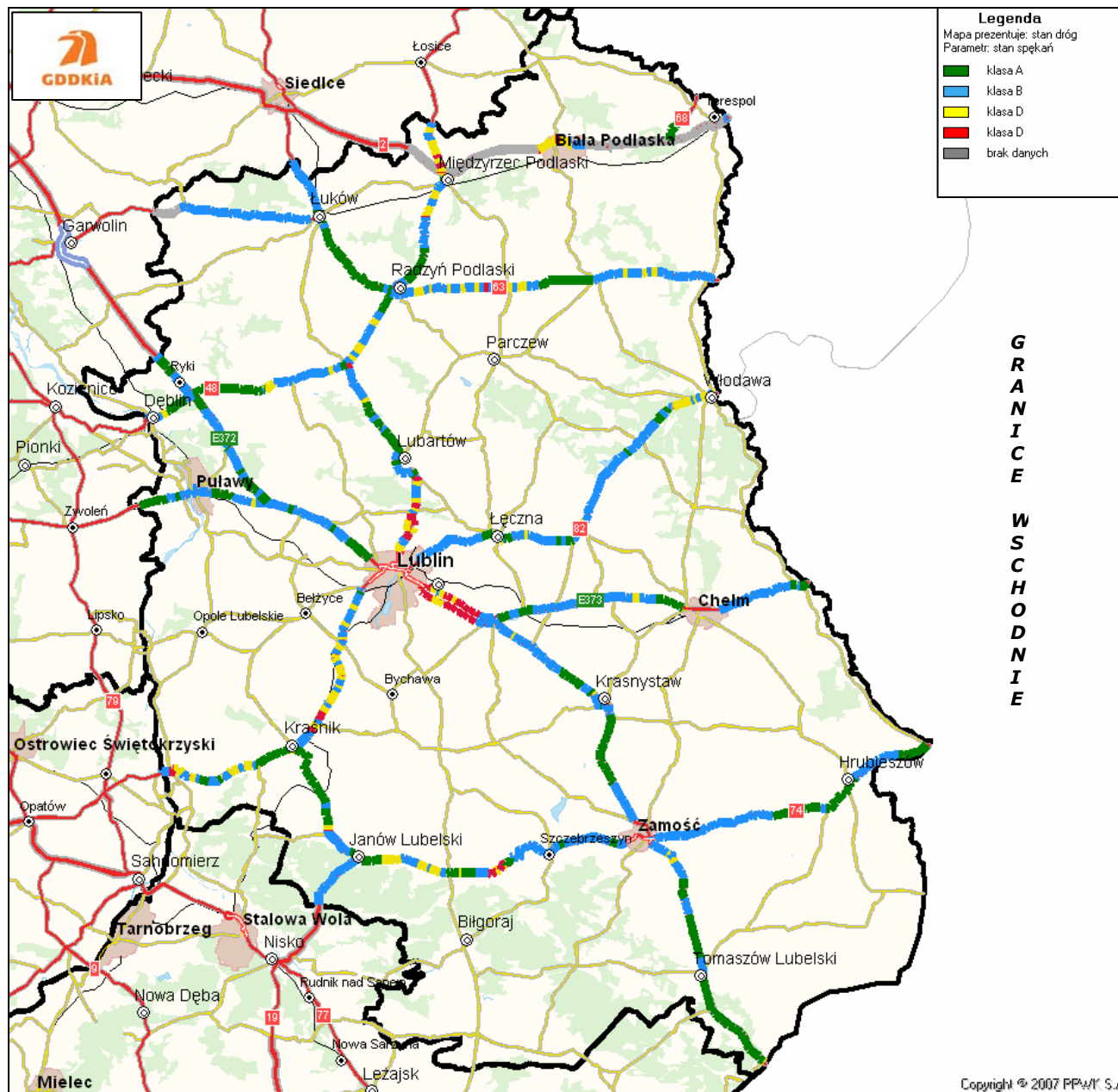
Rysunek 39. Lokalizacja odcinków ze stanem spekań w różnych klasach technicznych na terenie Oddziału w Lublinie
