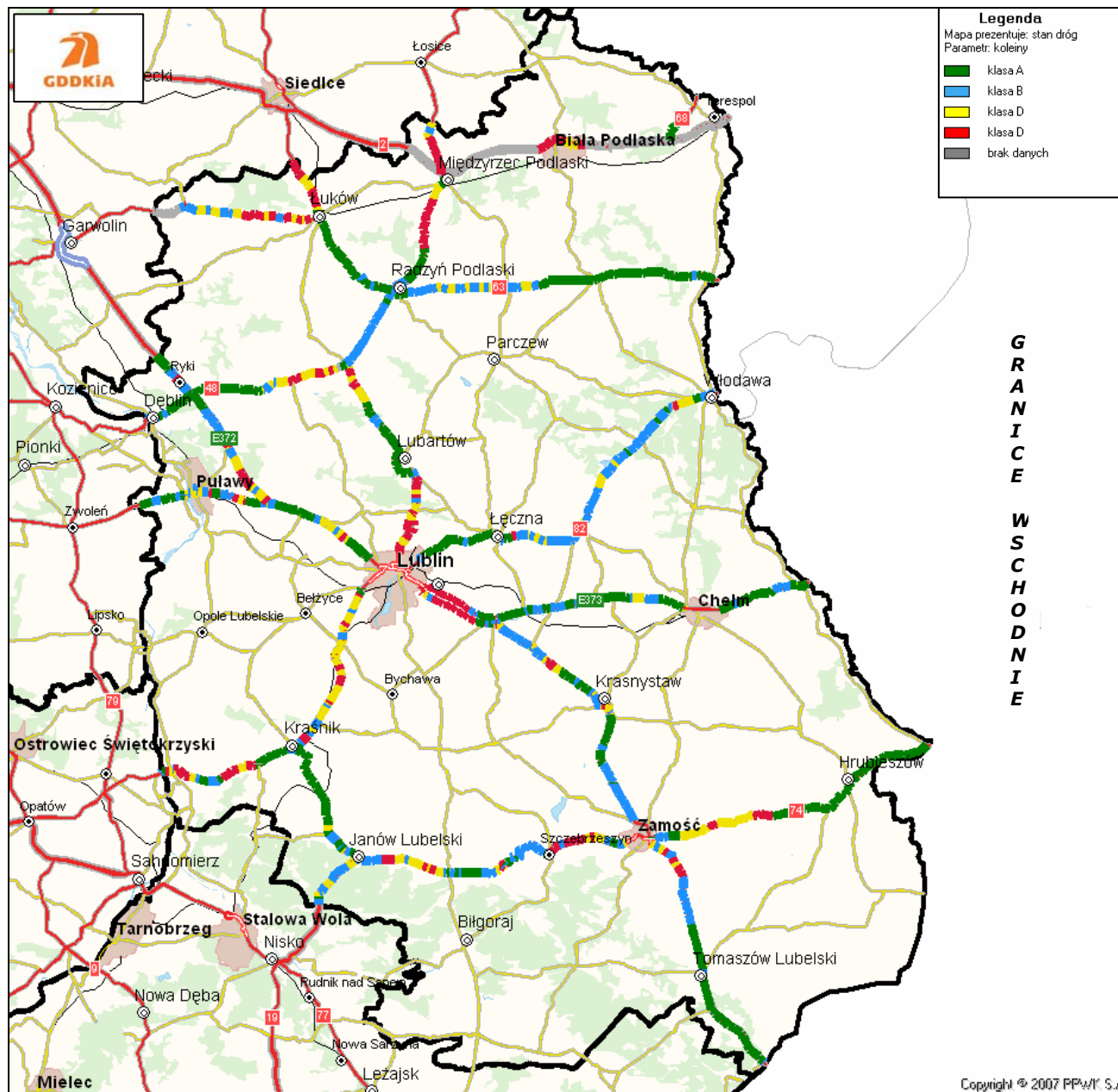
Rysunek 7. Lokalizacja odcinków z koleinami w różnych klasach technicznych na terenie Oddziału w Lublinie
