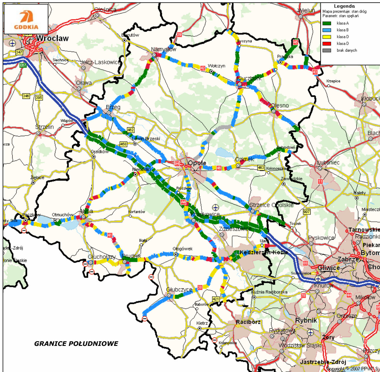
Rysunek 42. Lokalizacja odcinków ze stanem spełnień w różnych klasach technicznych na terenie Oddziału w Opolu
