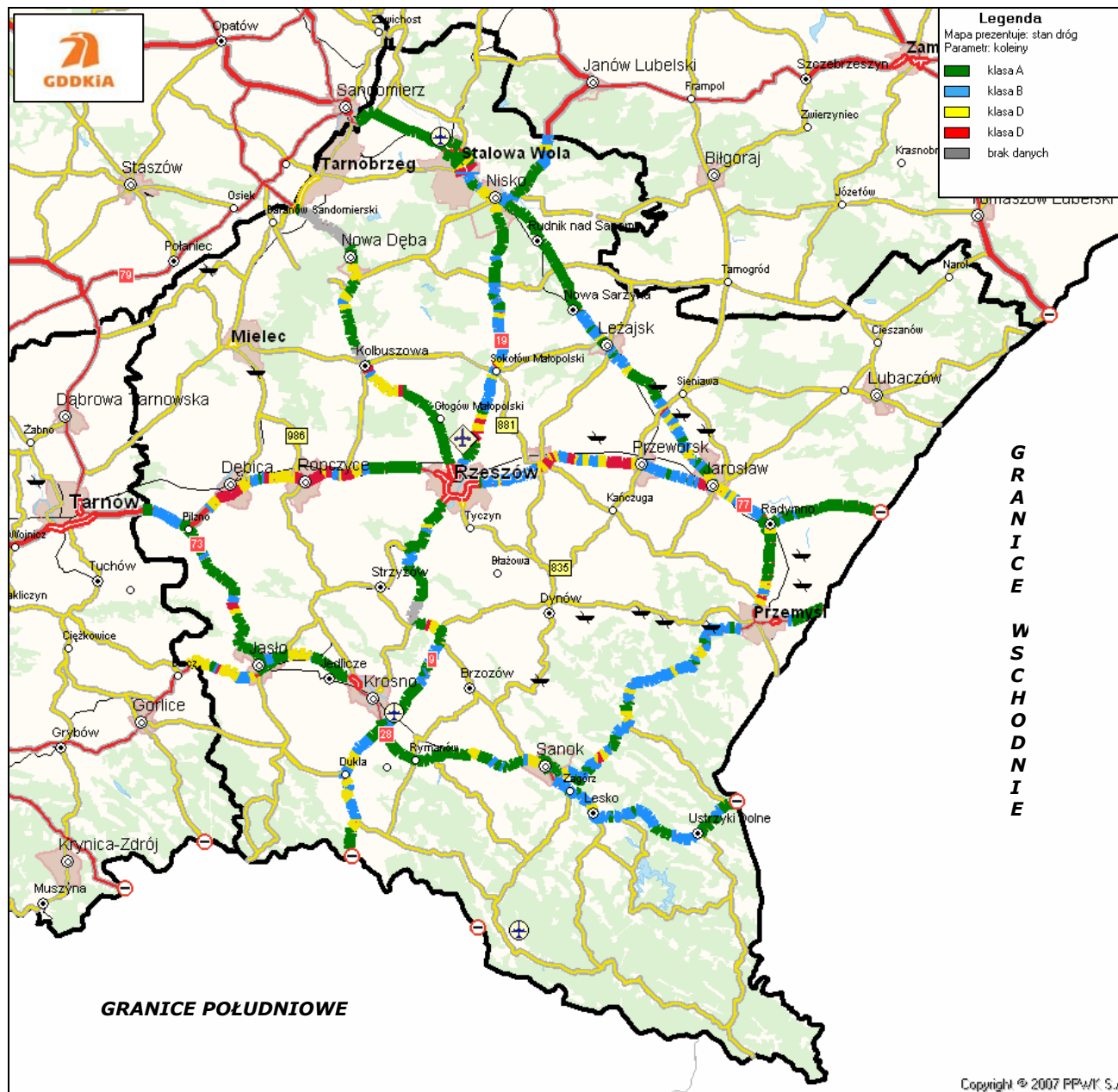
Rysunek 12. Lokalizacja odcinków z koleinami w różnych klasach technicznych na terenie Oddziału w Rzeszowie
