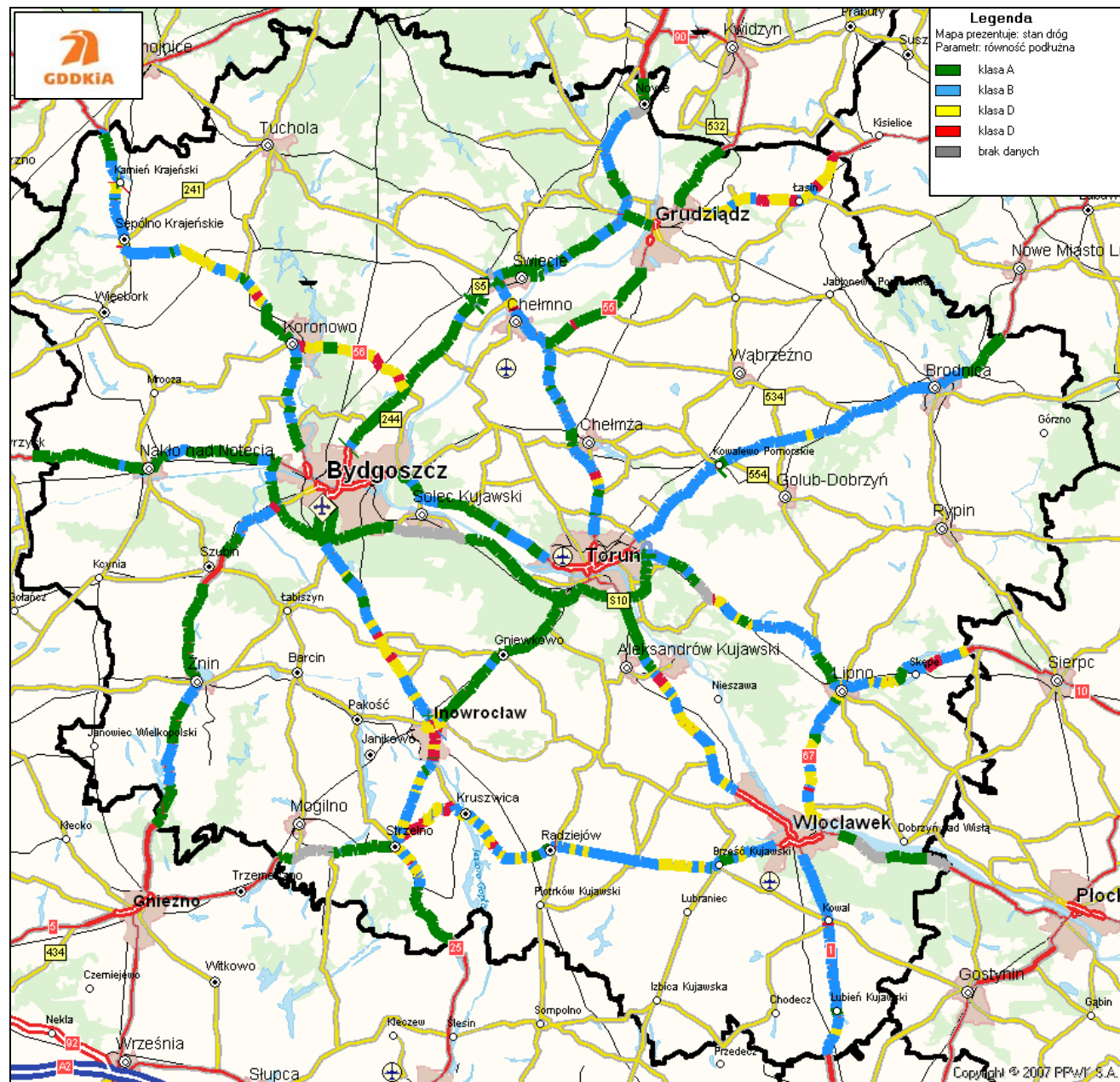
Rysunek 18. Lokalizacja odcinków z równością podłużną w różnych klasach technicznych na terenie Oddziału w Bydgoszczy
