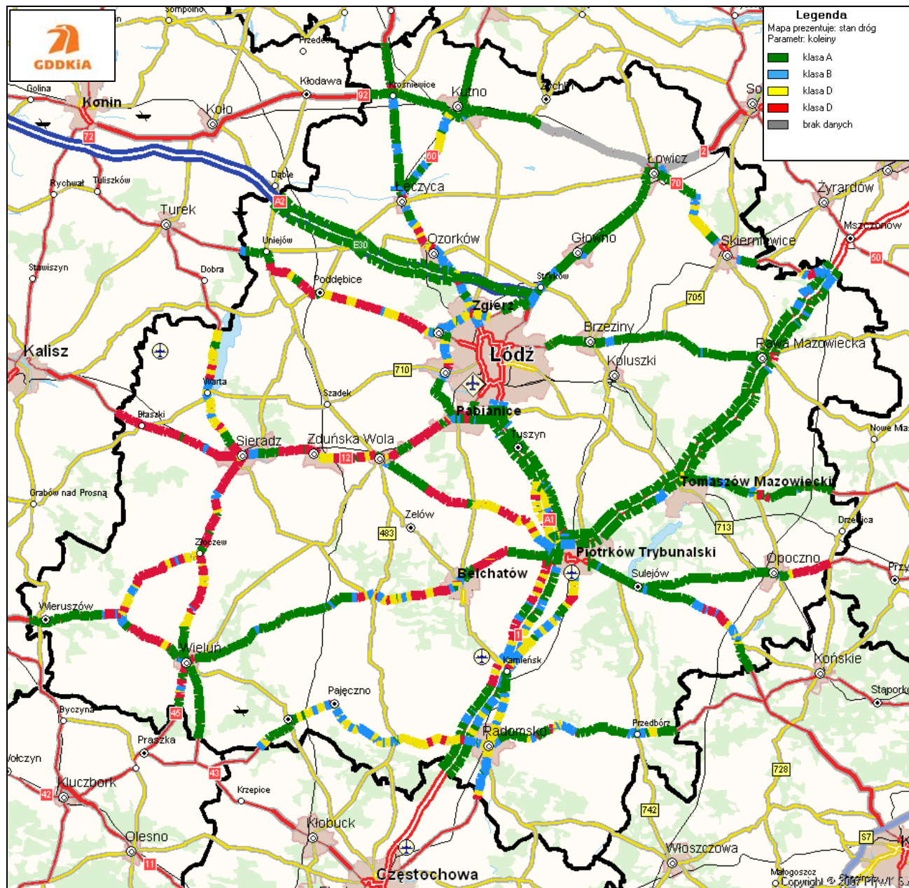
Rysunek 8. Lokalizacja odcinków z koleinami w różnych klasach technicznych na terenie Oddziału w Łodzi
