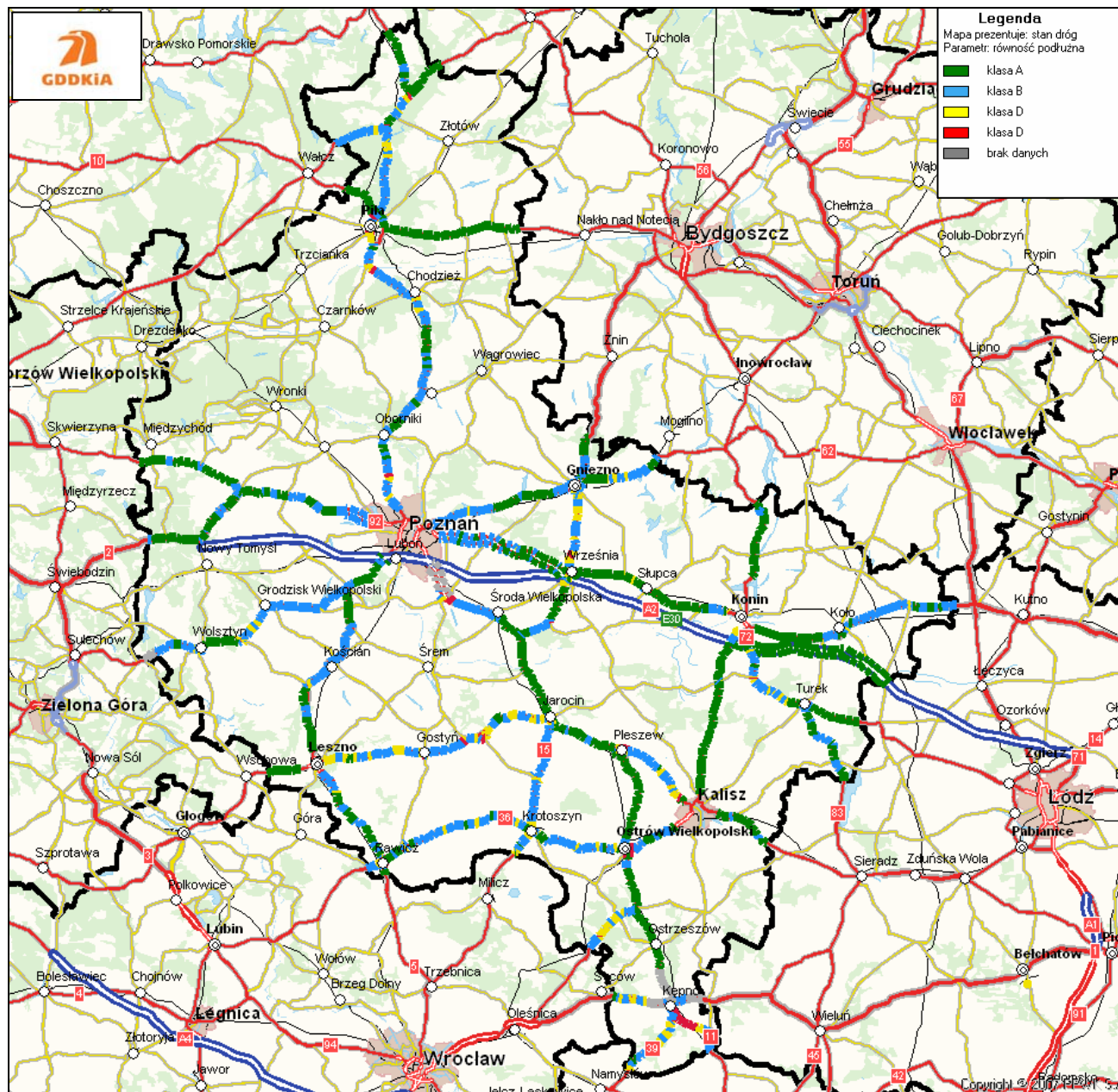
Rysunek 27. Lokalizacja odcinków z równością podłużną w różnych klasach technicznych na terenie Oddziału w Poznaniu
